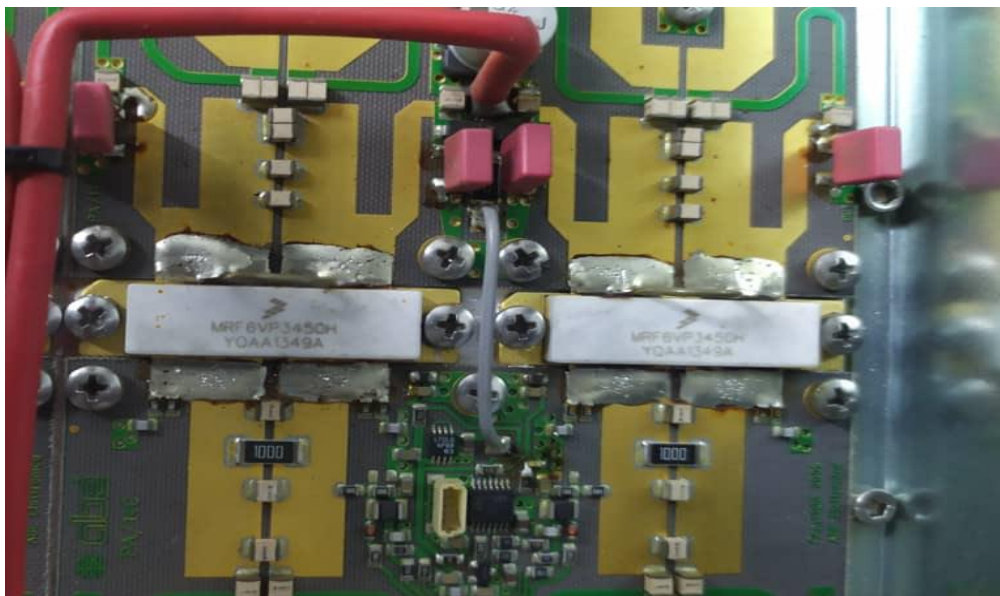
30-Module de carte d'amplificateur de puissance UHF 450W PA-14C avec transistor MRF6VP3450H
